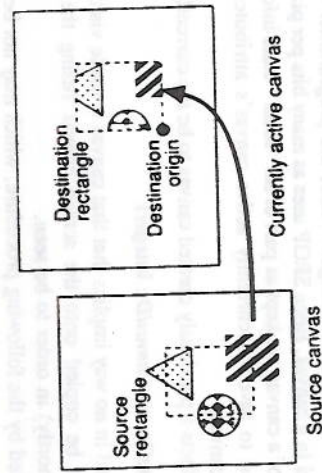
Fig. 2.26 SRGP_copyPixel.
