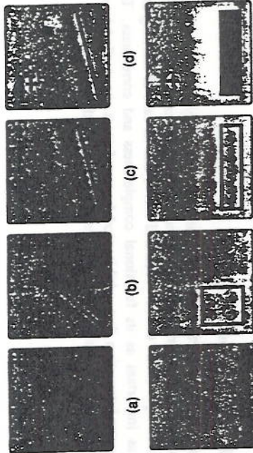
Fig. 2.23 Rubber-echo scenarios.
